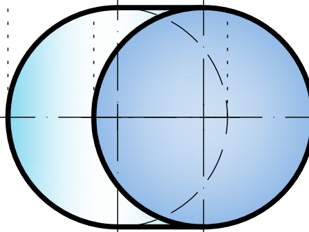
Cono oblicuo de vértice V_2 .
