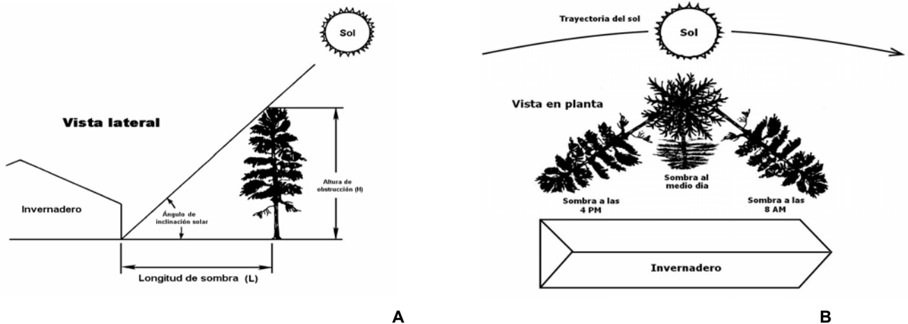
Figura 1.2.1 El cálculo del ángulo del sol en las diferentes estaciones del año es necesario para evitar sombras de objetos cercanos al invernadero (A). Las sombras incluso pueden cambiar de tamaño y posición durante el día (B). (modificado de Walker y Duncan, 1974).
