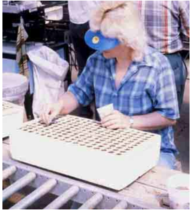
Figura 1.4.26. La sembradora de vacío (A) succiona las semillas y las retiene en la oquedad que coincide con el mismo patrón de la rejilla y las celdas del contenedor. El número de cavidades determina la densidad de siembra (B). Cuando el vacío se interrumpe, el contenedor es sembrado completamente de una sola vez (C). Tanto la caja perforada con rejilla móvil como la sembradora de vacío requieren supervisión, y a menudo se necesita semilla extra para sembrarla en cavidades vacías (D).
