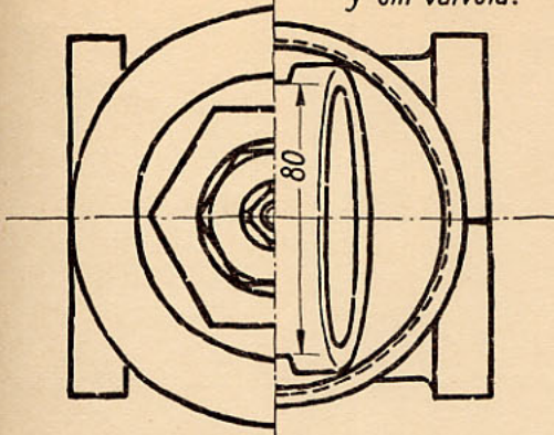
Semi proyección sin tapa y sin válvula.
